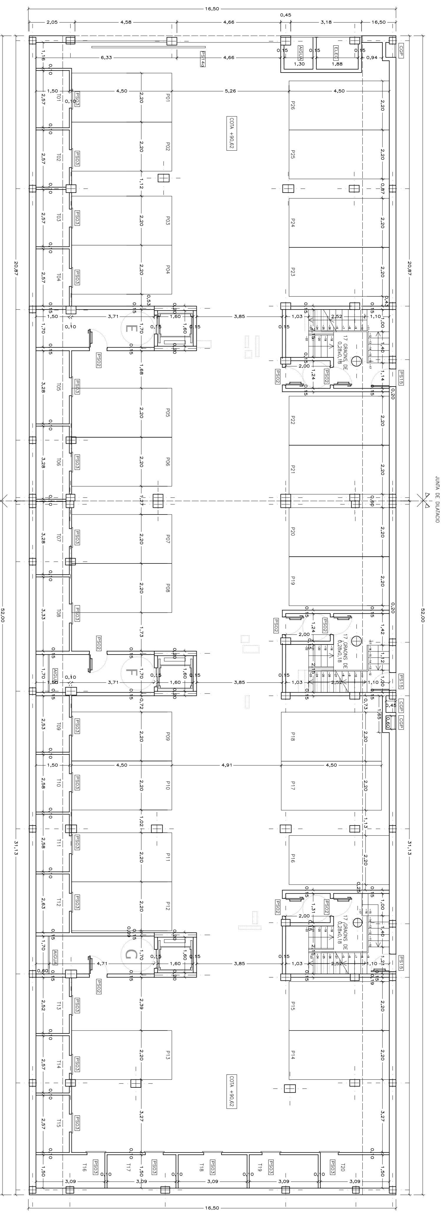
PLANTA SOTERRANI-1 SUPERFÍCIE CONSTRUIDA 855,92m 2 (NO COMPUTABLE)
